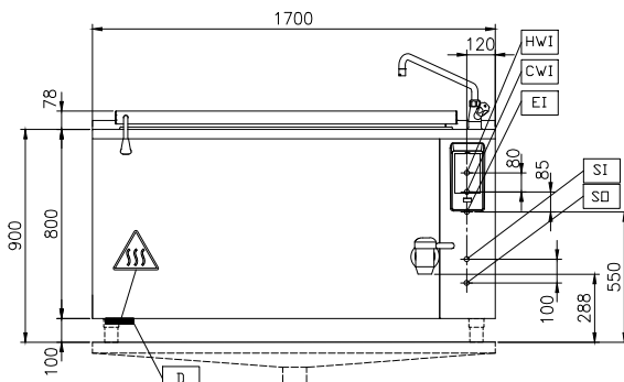
Front aanzicht
